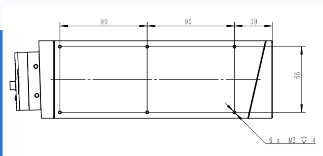
底面图（安装定位孔）
