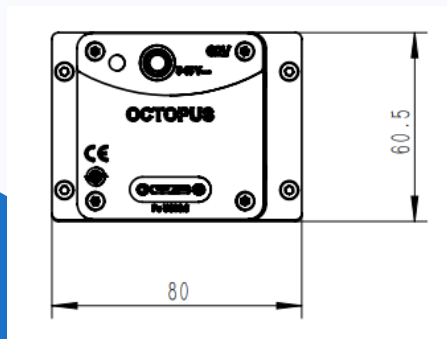
侧面图
